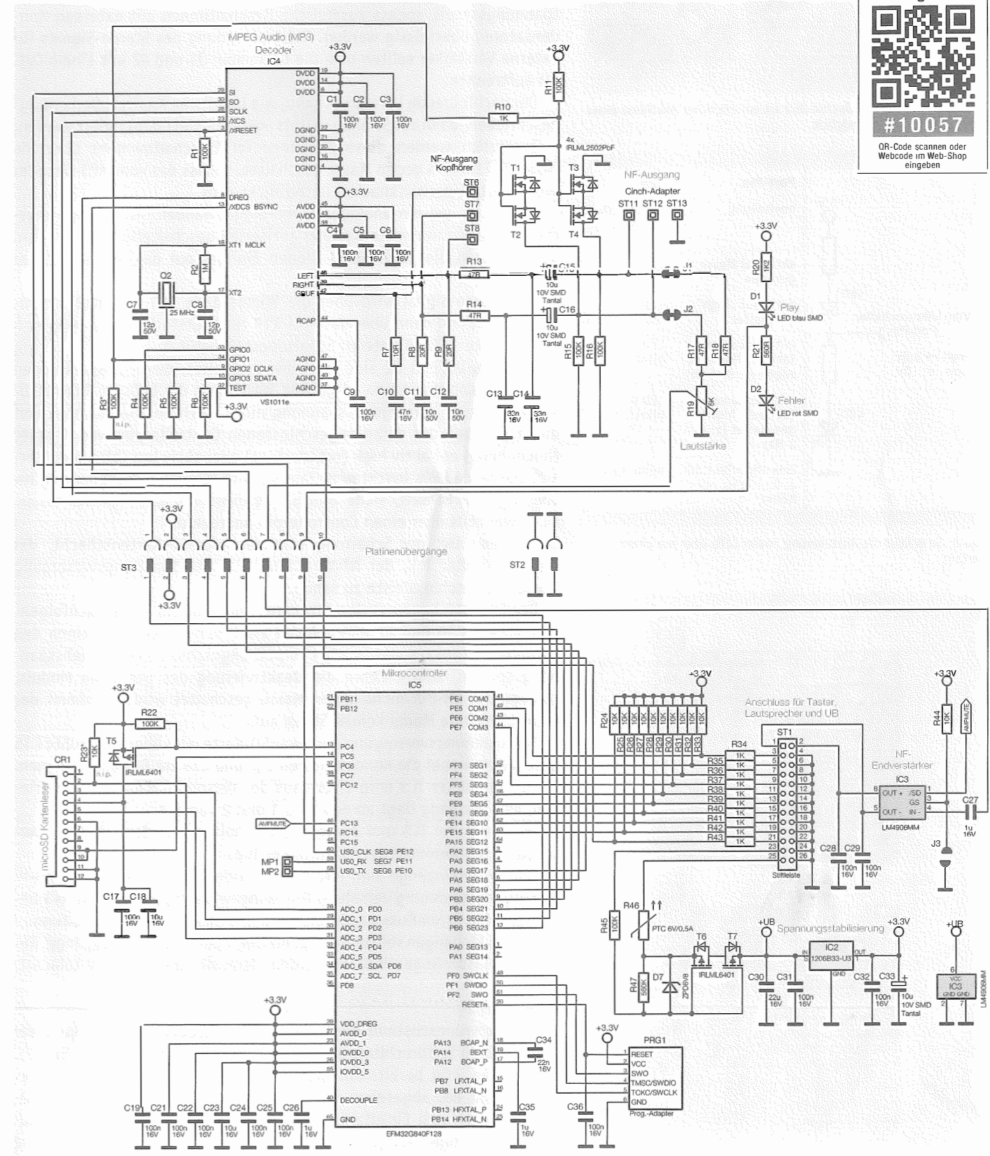
Bild 4: Das Schaltbild des MSM4
