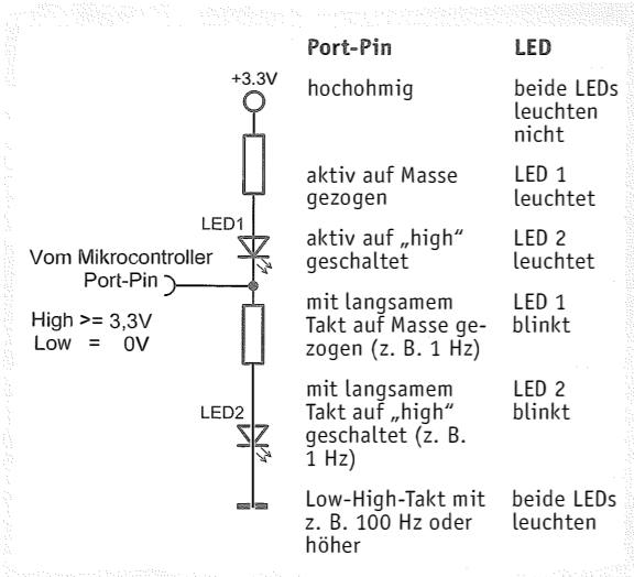
Bild 6: So erfolgt die Ansteuerung zweier LEDs über nur einen Portpin.
