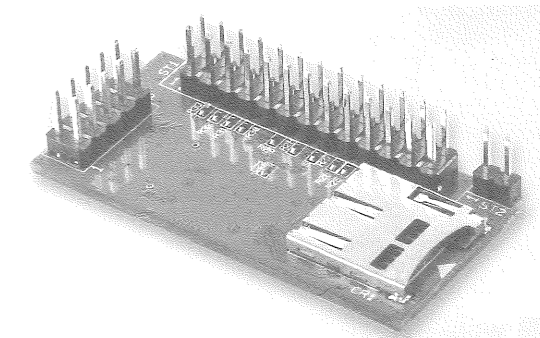
Bild 9: Die mit den Stiftleisten bestückte Platine des MSM4
