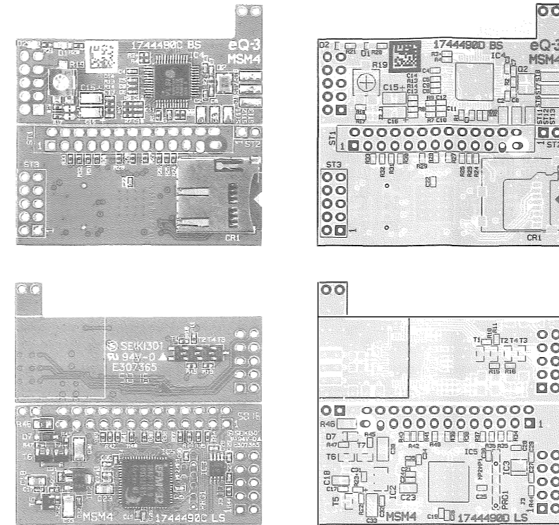
Bild 8: Die Platinenfotos mit den zugehörigen Bestückungsplänen für die MP3-Player-Platinen und die Cinch-Adapterplatine
