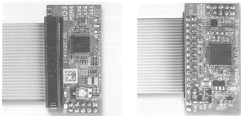
Bild 11: Sämtliche Anschlüsse des MP3-Soundmoduls können über einen Flachbandkabel-Steckverbinder hergestellt werden.
